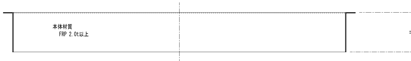
A~A' 断面
